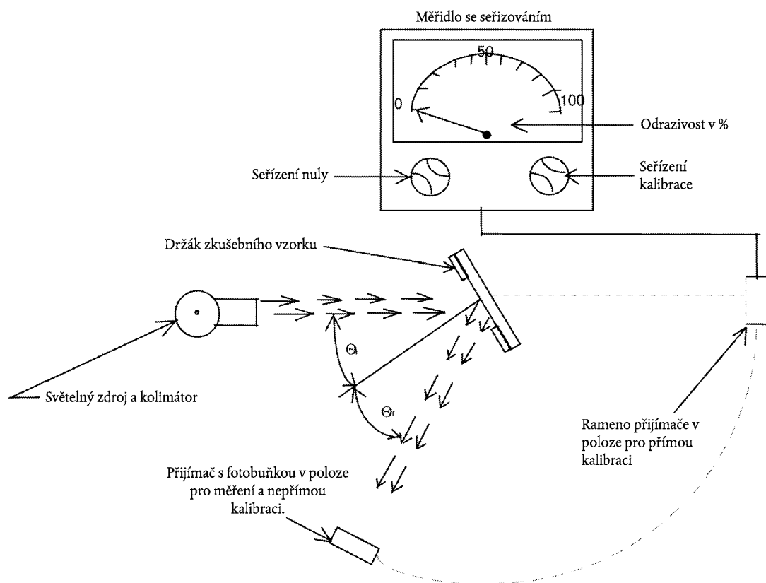
Obrázek 4: Zobecněné schéma reflektometru se znázorněním seřízení pro dvě kalibrační metody
