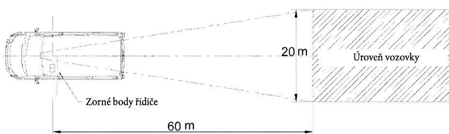
Obrázek 6: Pole výhledu zrcátek třídy I
