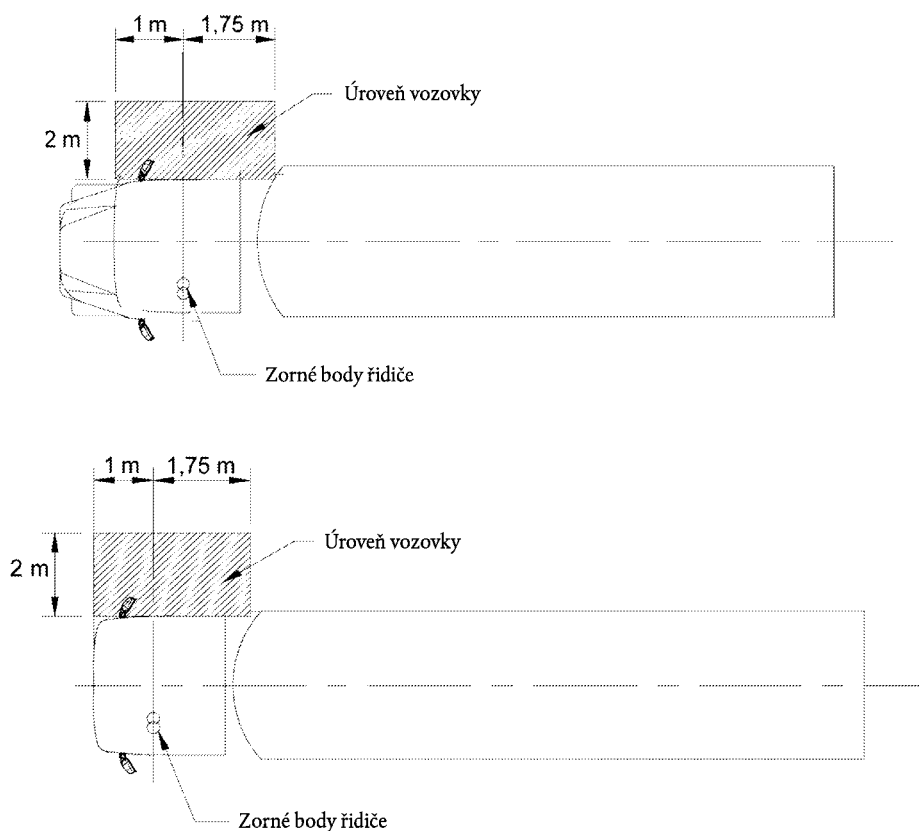
Obrázky 10a a 10b: Pole výhledu u blízkopohledových zrcátek třídy V
