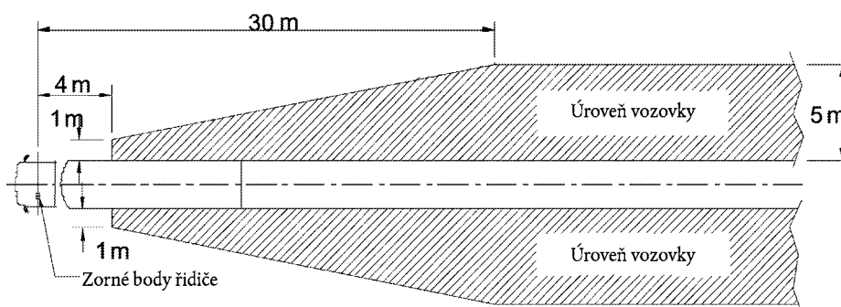
Obrázek 7: Pole výhledu zrcátek třídy II
