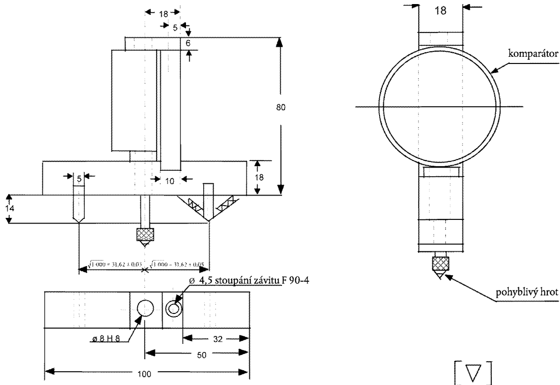
Obrázek 3: Sférometr
