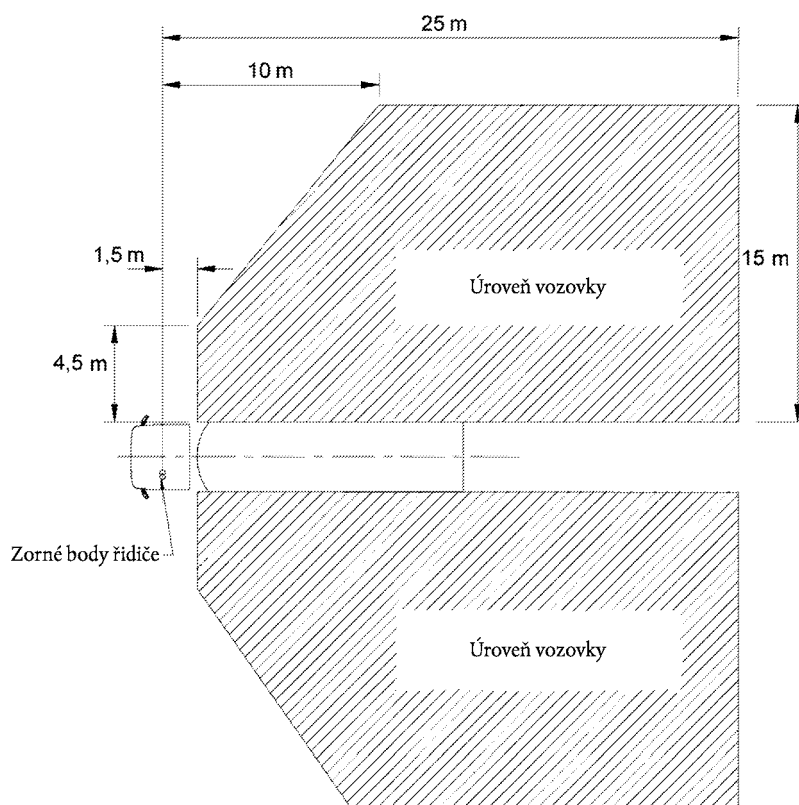
Obrázek 9: Pole výhledu širokoúhlých zrcátek třídy IV
