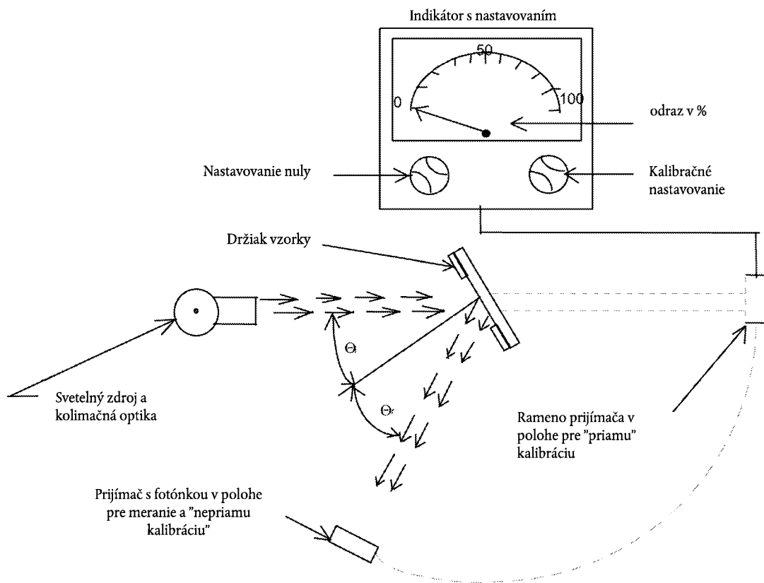
Obrázok 4: Všeobecná schéma reflektometra s vyznačením oboch kalibračných metód
