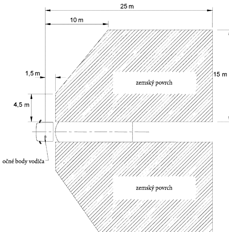
Obrázok 9: Výhľad poskytovaný širokohlým zrkadlom triedy IV
