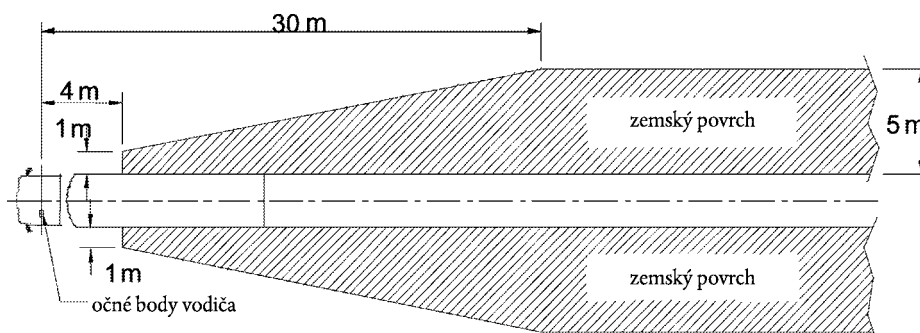
Obrázok 7: Výhľad poskytovaný zrkadlom triedy II
