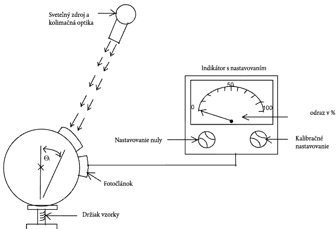
Obrázok 5: Všeobecná schéma reflektometra s Ulbrichtovou guľou v prijímači
