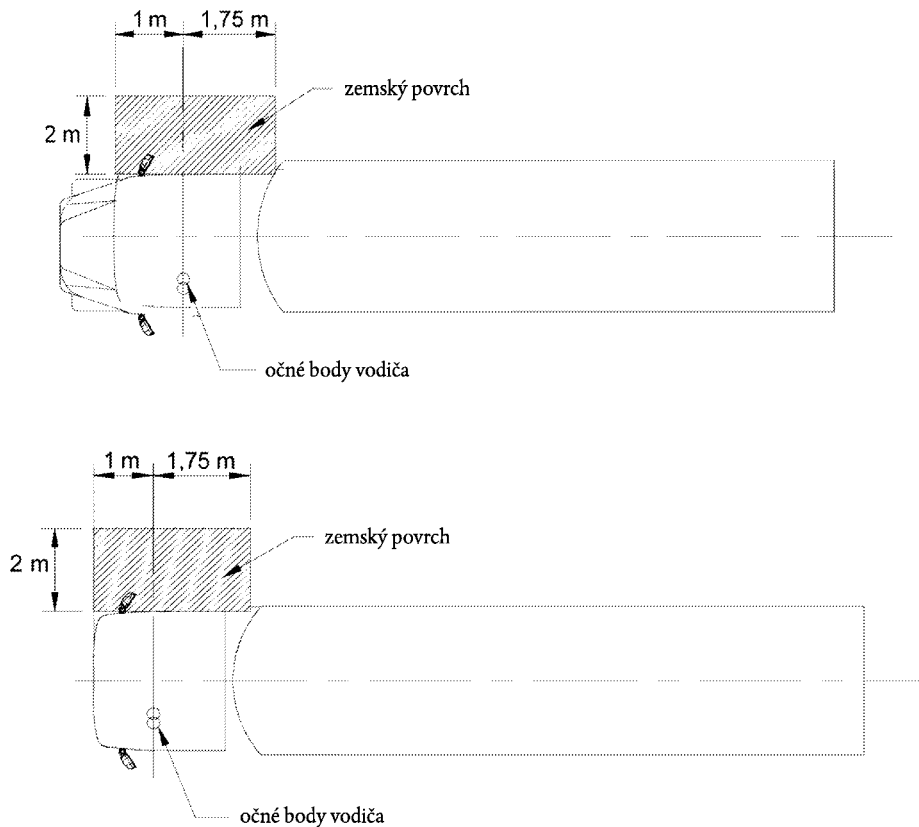
Obrázky 10a a 10b: Výhľad poskytovaný blízkovýhľadovým zrkadlom triedy V
